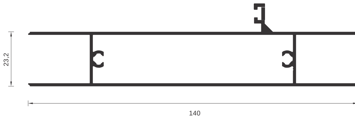
BATENTE PORTA PIVOTANTE
